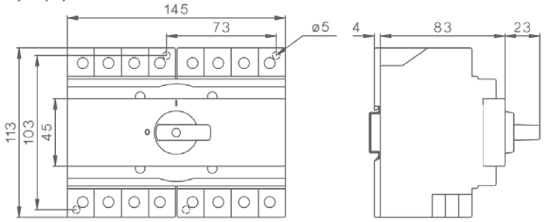
SI40DB(L) / SI55DB(L) / SI65DB(L)
