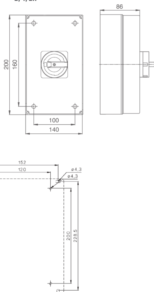
SI40PEL / SI55PEL / SI65PEL 2, 4, 2H
