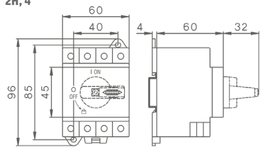
SI40DB(L) / SI55DB(L) / SI65DB(L)
