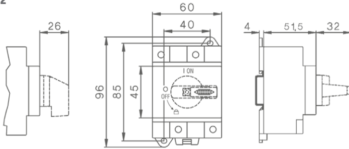
SI40DB(L) / SI55DB(L) / SI65DB(L)
